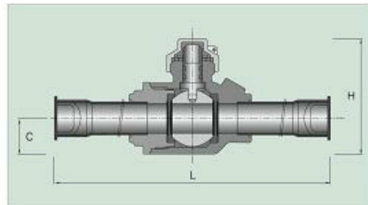
Schraeder szelep nélküli verzió
