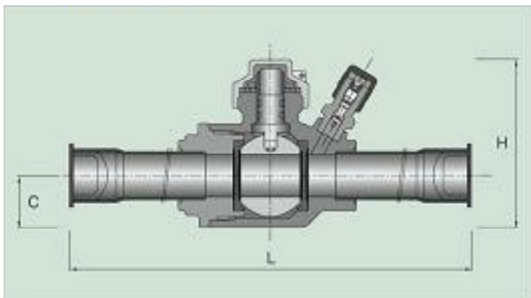
Schraeder szelepes verzió
